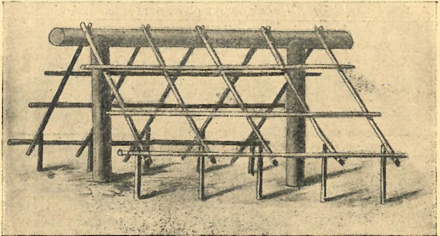
26. sz. ábra. Napvédő váza.
