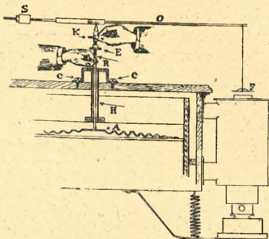
19. sz. ábra. A legújabb Kogler- és Roszner-féle magyar gyártmányú keltetőgép önszabályozójának szerkezete.
