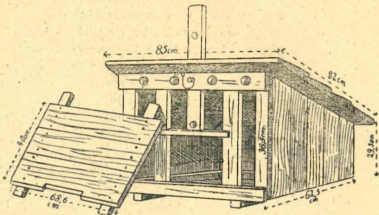
21. sz. ábra. Pulykakotlóborító.
