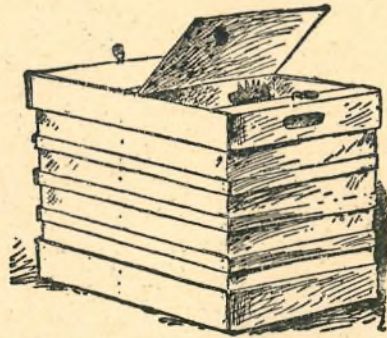
43. sz. ábra. Tenyézpulykaszállító rekesz.
