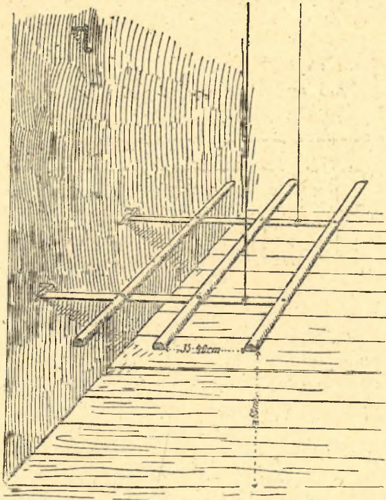
35. sz. ábra. Felhuzható ülőrud-szerkezet.
