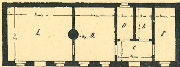
31. sz. ábra. A pulykaház belső beosztása.
