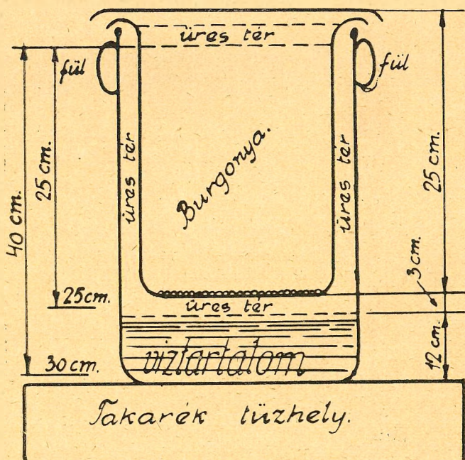
A burgonyapároló készülék vázlatrajza.
